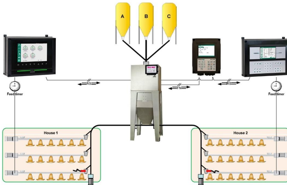
Overzichtsschema
