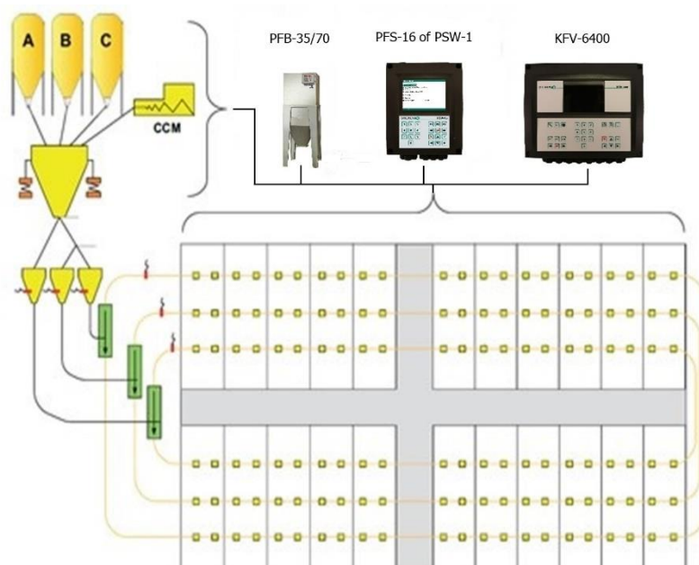
Overzichtsschema
