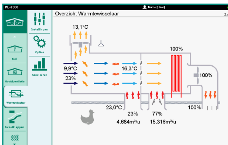
overzicht warmtewisselaar
