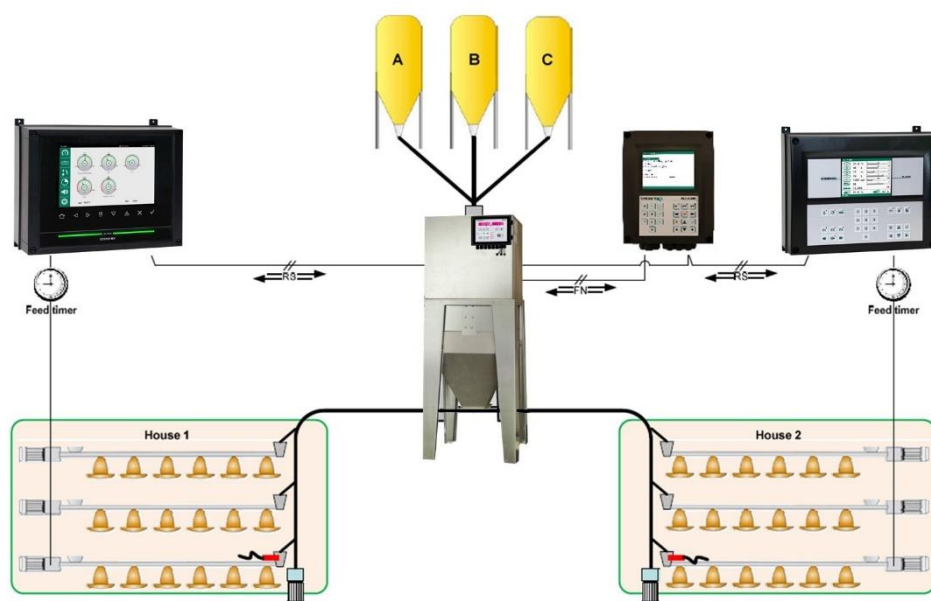
Overzichtsschema
