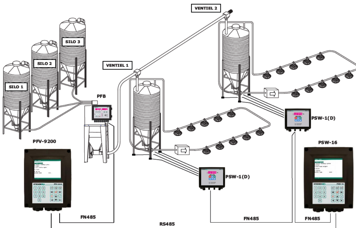
Overzichtsschema
