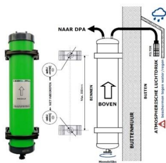
Optioneel: RPF-01 Referentie drukfilter
