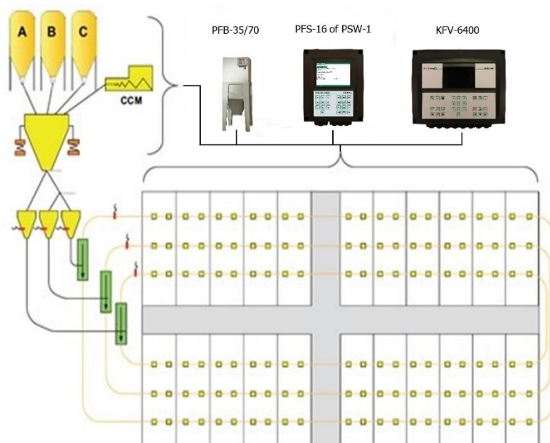
Overzichtsschema
